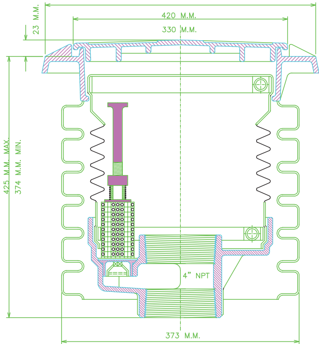
ARQUETA ANTIDERRAME
